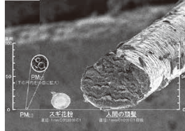
PM2.5 の大きさのイメージ (東京都 HP から引用)
