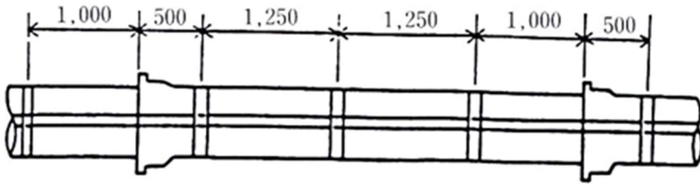
図-2 6 m管
