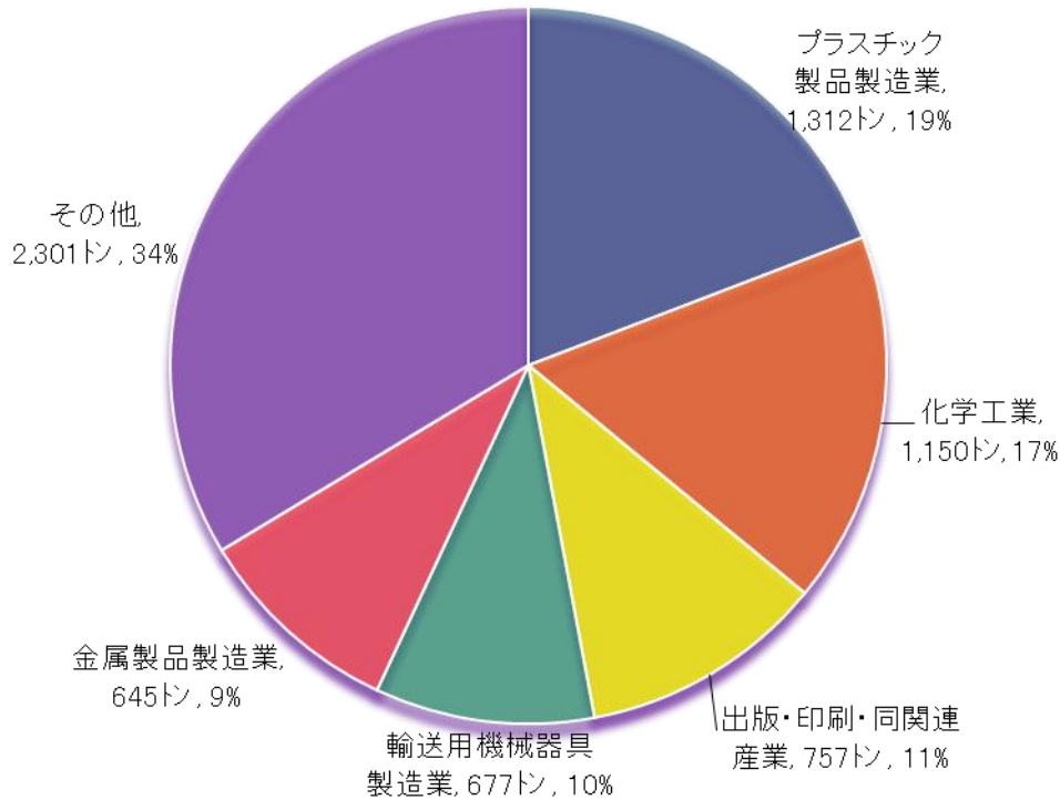
図2. 埼玉県の業種別の届出排出量と構成比
