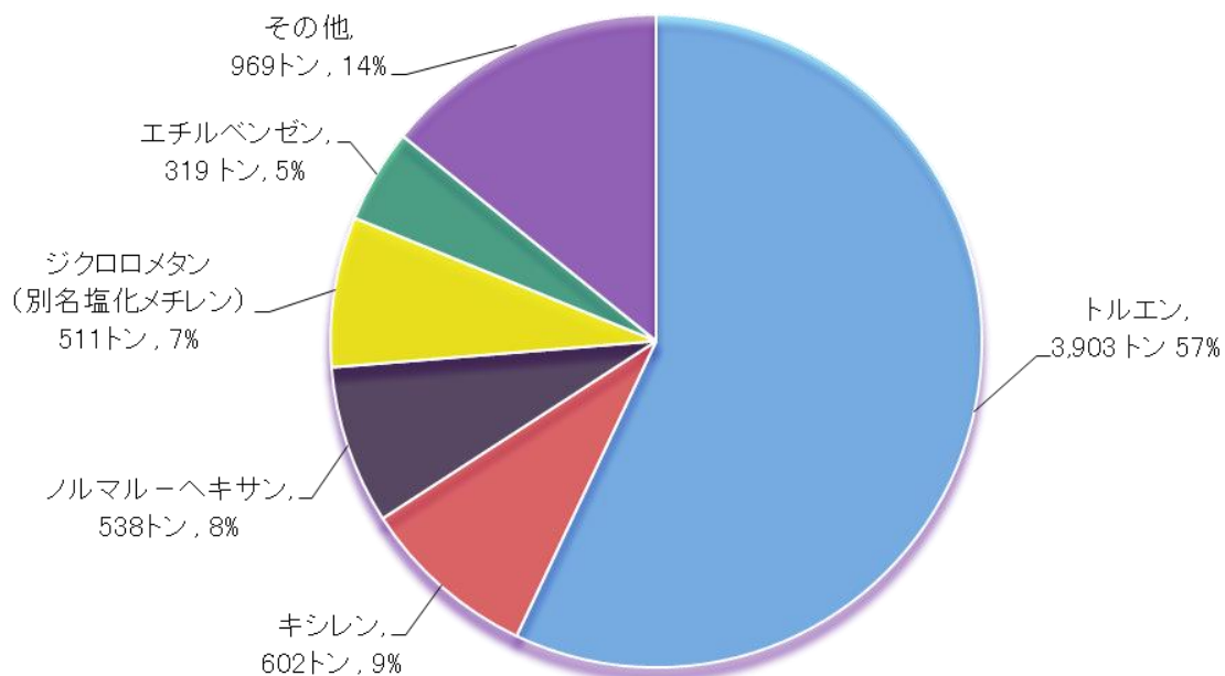
図 1. 埼玉県の物質別の届出排出量と構成比
