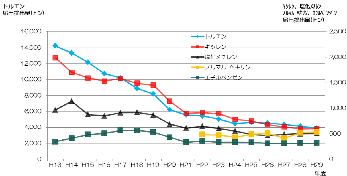
図4 埼玉県届出排出量上位5物質の排出量の経年変化
