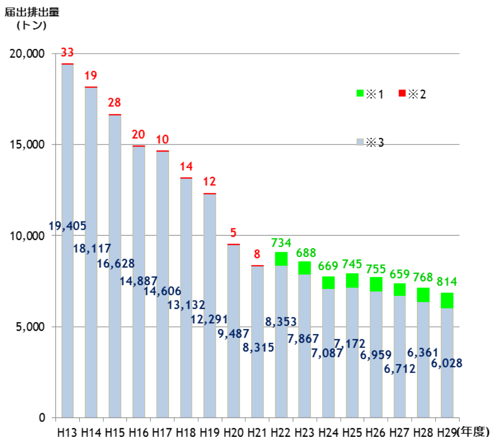
図3 埼玉県 の届出排出量の経年変化
