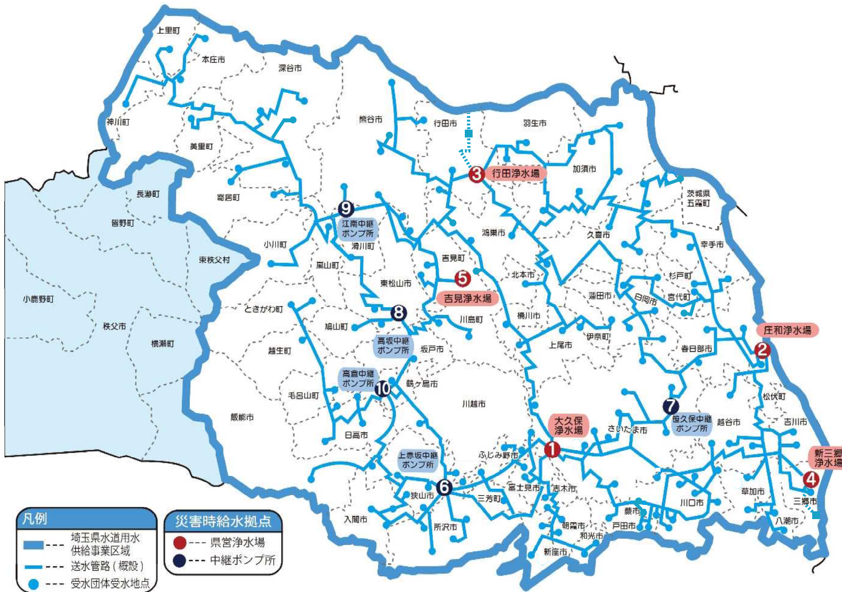
(図) 埼玉県水道用水供給区域図 (浄水場・中継ポンプ所・送水管路・災害時給水拠点)
