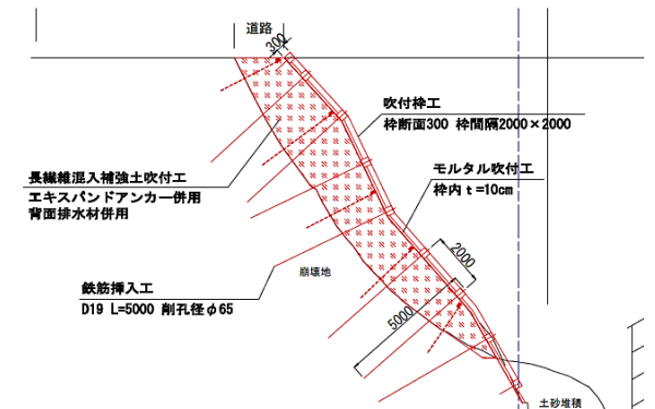
対策標準断面
