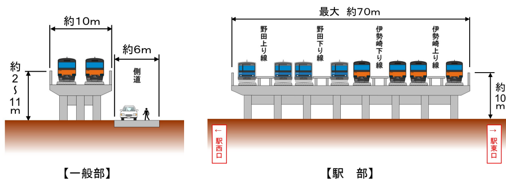
横断面図（イメージ）
