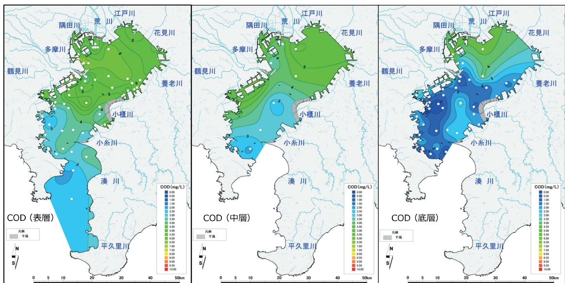
図 5-4 令和 4 年 8 月 3 日における東京湾の COD の状況
