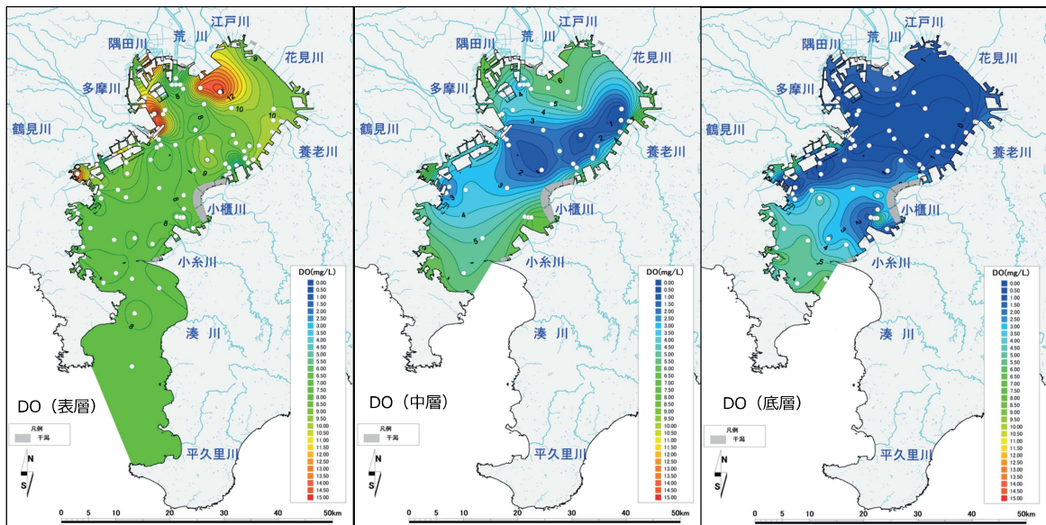
図 5-3 令和 4 年 8 月 3 日における東京湾の DO の状況
