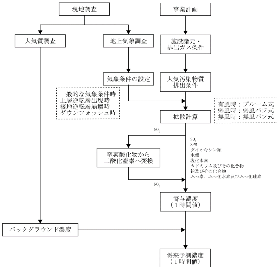
図 9.1-17 施設の稼働に伴う予測手順（短期高濃度（１時間値））
