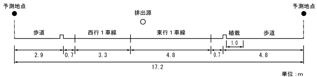
図 9.1-15 道路断面図
