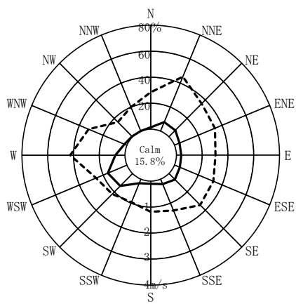
図 9.1-4(5) 風配図（4季：No.4）
