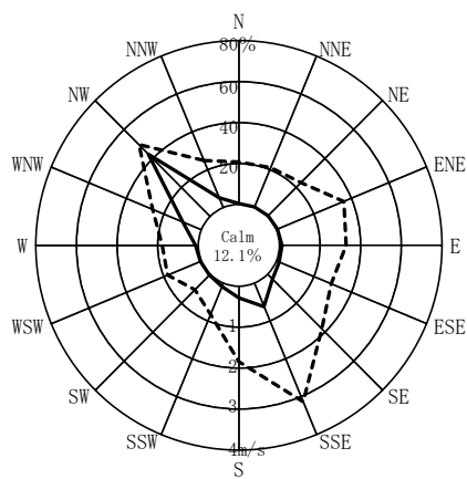
図 9.1-4(1) 風配図（4季：地点A）
