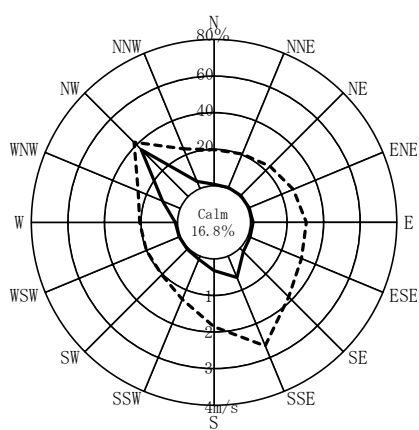
図 9.1-3 風配図（通年）
