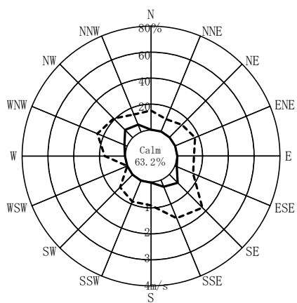
図 9.1-4(3) 風配図（4季：No.2）
