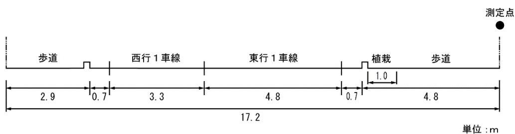
図 9.2-3 道路断面図
