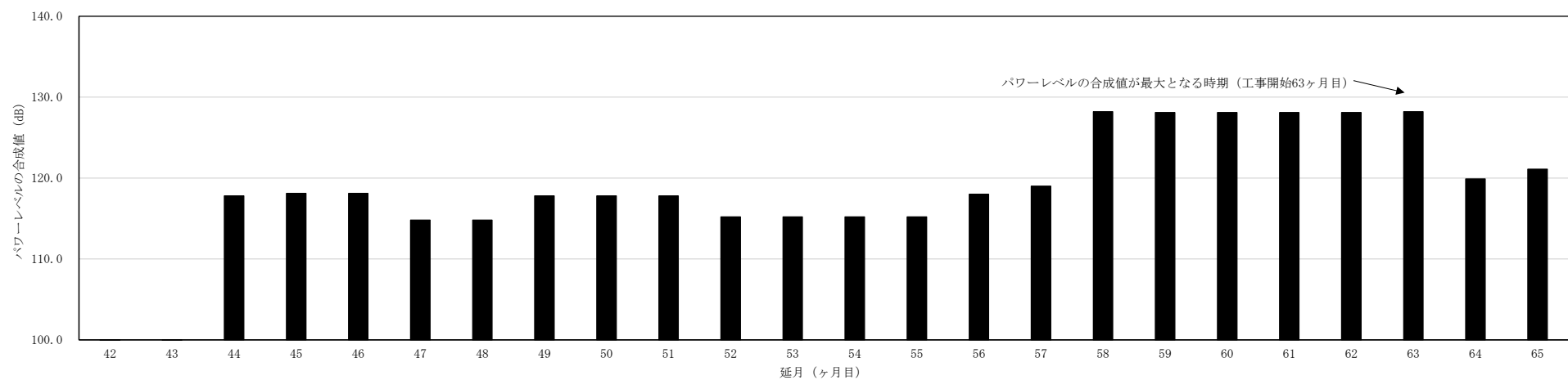
図 4. 2-1 (2) 建設機械の稼働に伴うパワーレベルの合成値の推移（既存施設解体工事）
