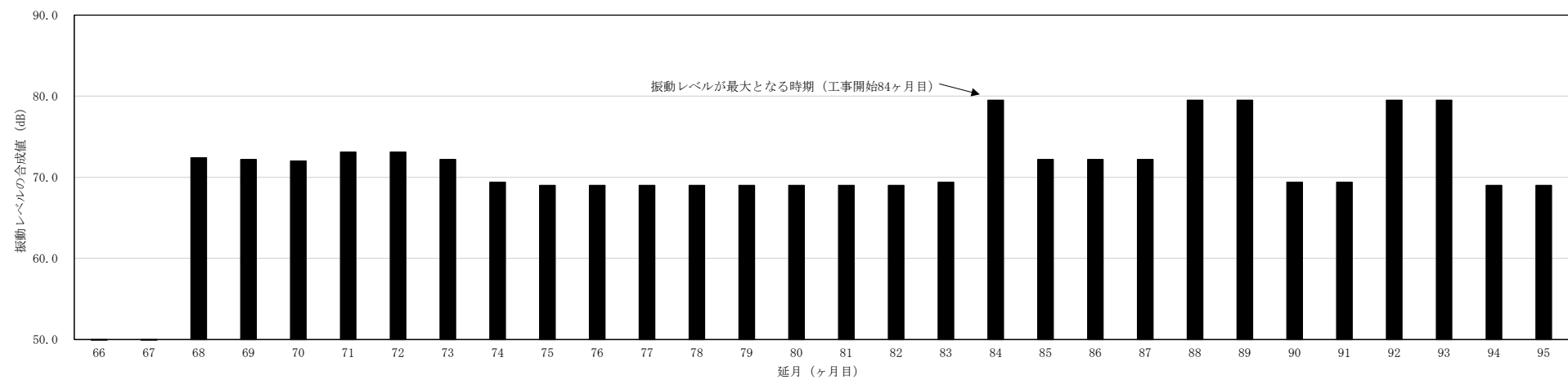
図 5.2-1 (3) 建設機械の稼働に伴う振動レベルの合成値 (Ⅱ期工事)
