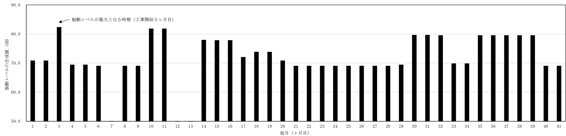
図 5. 2-1 (1) 建設機械の稼働に伴う振動レベルの合成値 (I 期工事)
