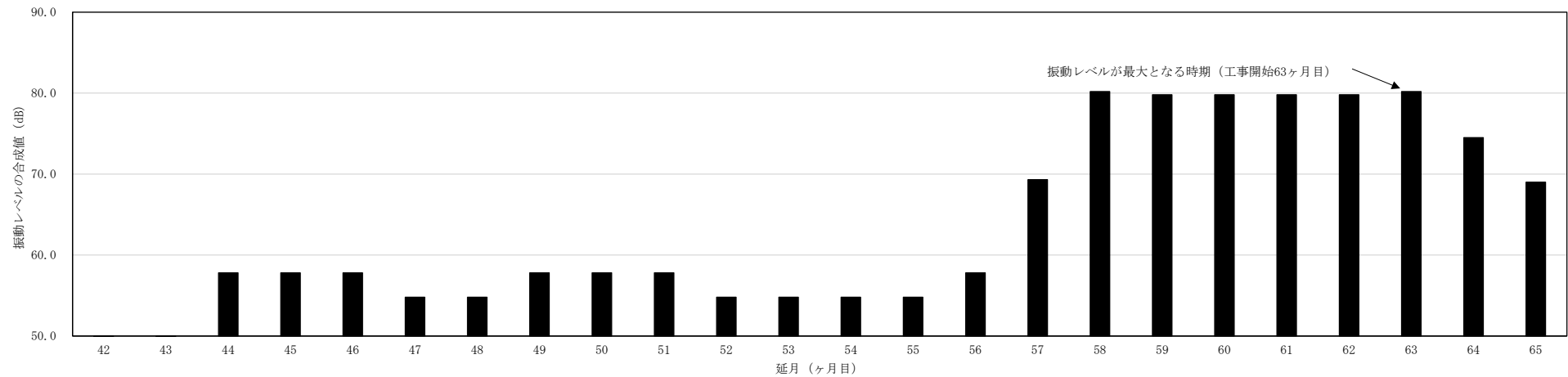
図 5. 2-1 (2) 建設機械の稼働に伴う振動レベルの合成値 (既存施設解体工事)
