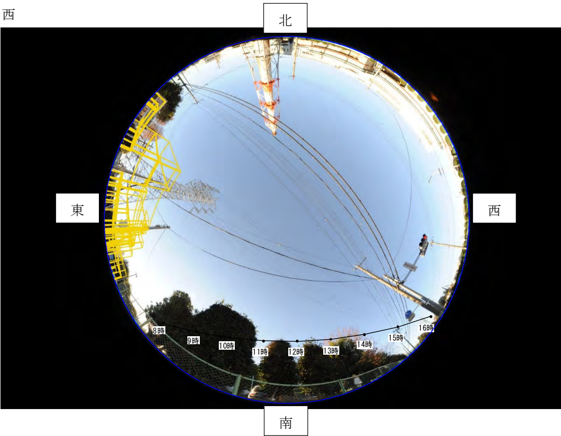
図 9-11-8(1) 天空図(8 時)
