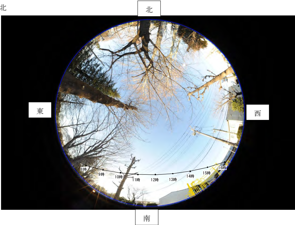
図 9-11-8(2) 天空図(8 時)
