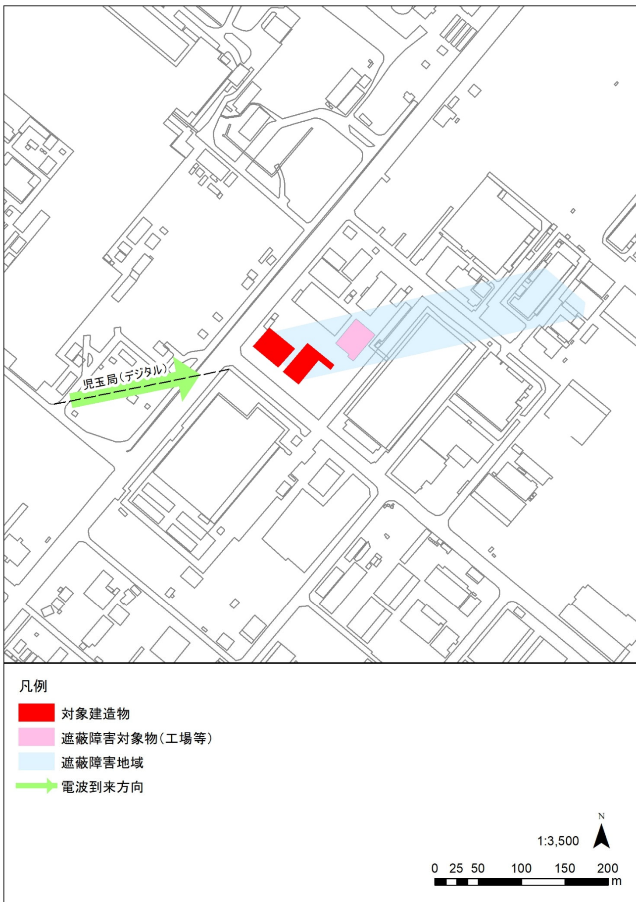
図 9-12-1 電波障害の予測範囲（地上デジタル放送（児玉局））
