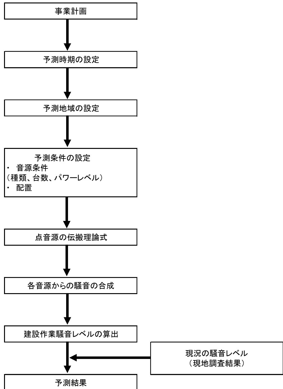
図 9-2-3 建設機械の稼働に伴う建設作業騒音レベルの予測手順
