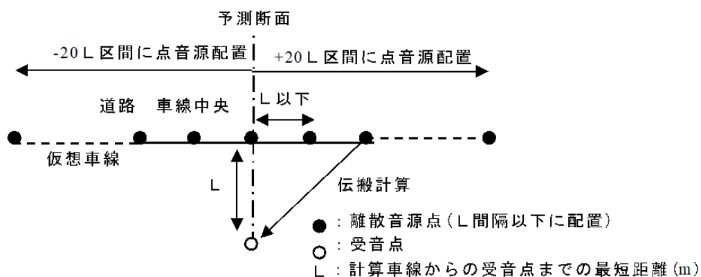
図 9-2-7 音源配置図 (道路延長方向の配置イメージ)
