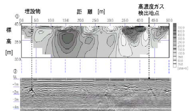
図3-16 ①比抵抗構造断面と②地中レーダプロフィール
