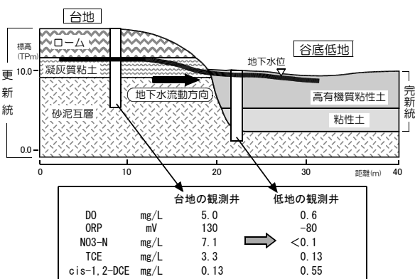
図3-13 TCE汚染地下水の地下水流動と還元反応
