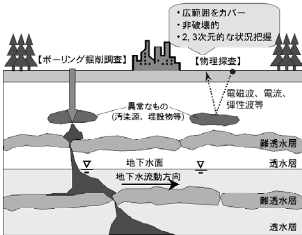
図3-15 汚染調査における物理探査の概念図
