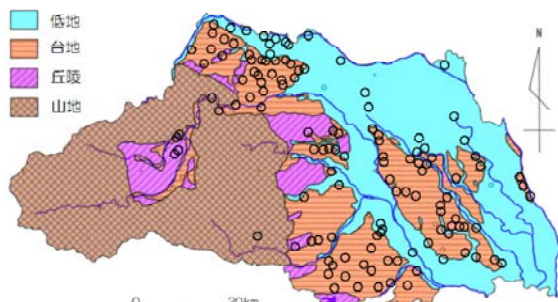
図3-11 硝酸・亜硝酸性窒素による汚染井戸分布
