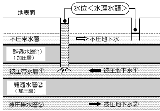
図2-5 地下水の存在形態の模式図
