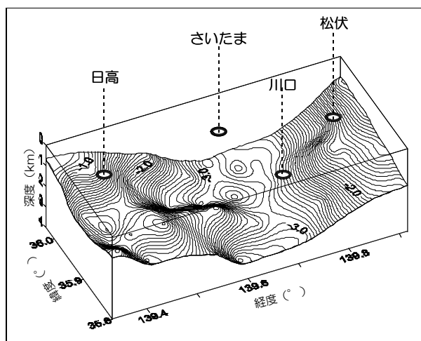
図4-8 県南部平野の3次元基盤形状 21)
