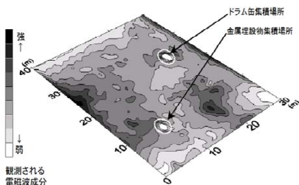
図3-17 地表面付近の電磁波成分の分布
