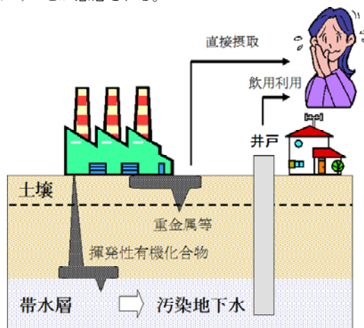
図3-2 市街地土壌汚染と有害物質の暴露経路
