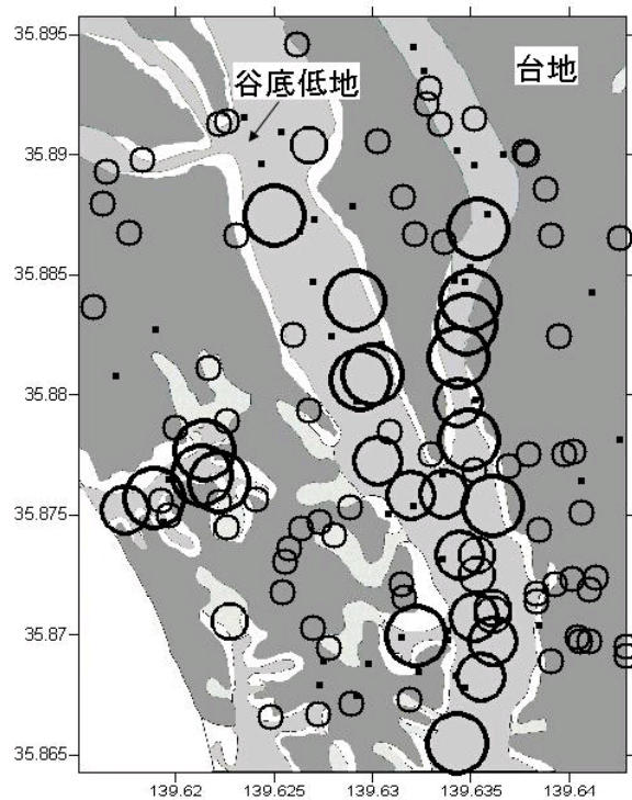
図4-9 地形による増幅度の違い
