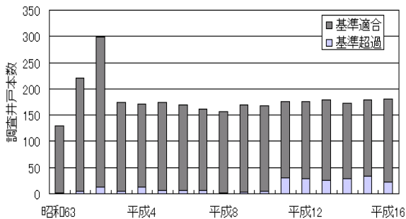
図3-9 地下水質概況調査結果の推移
