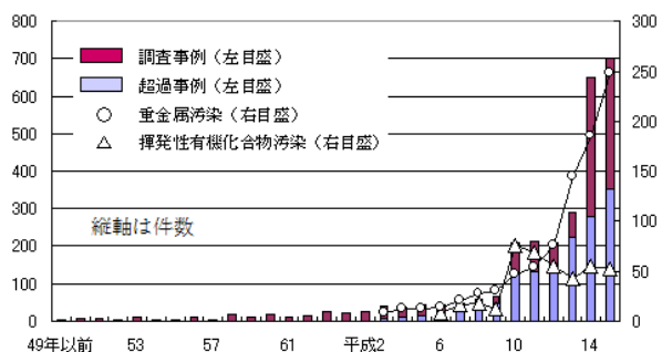
図3-3 土壌汚染判明件数の推移 11)
