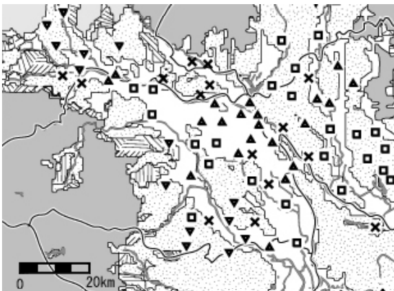
図2-9 地下温度プロファイルに基づく関東地下水盆の地下水涵養域と流出域の分布 9) (▼:涵養域型、□:中間域型、▲:流出域型、×:その他)
