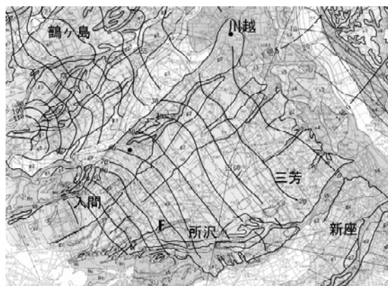
図2-7 武蔵野台地北部における浅層地下水面の分布 7)
