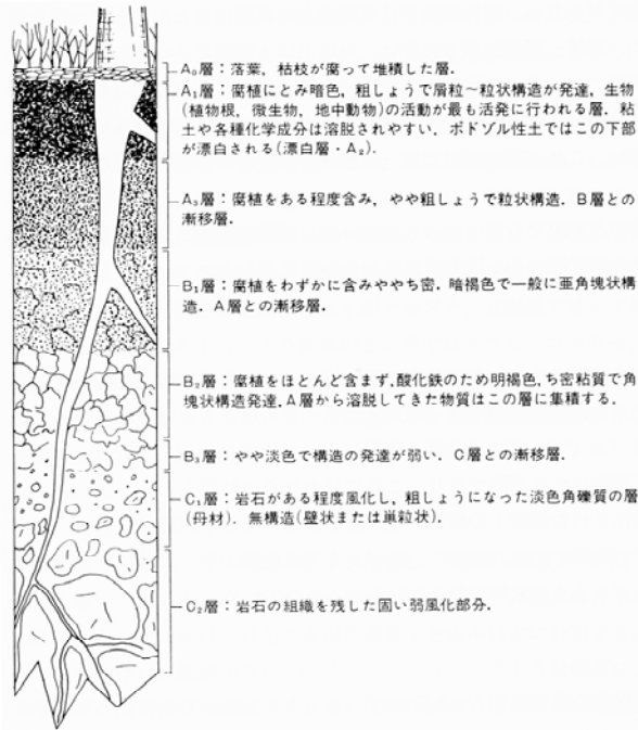
図2-3 土層断面の構成と土層層位の特徴 3)
