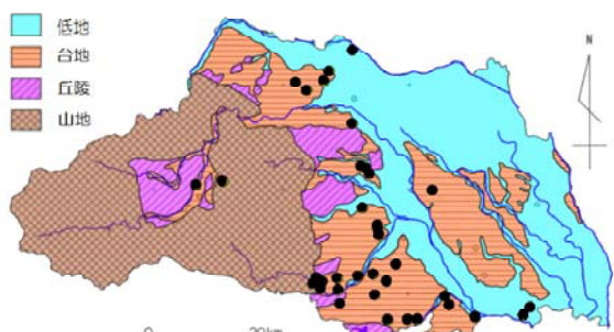
図3-12 TCE及びPCEによる汚染井戸分布
