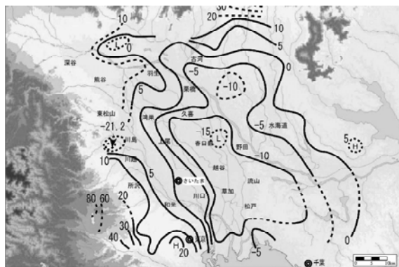
図2-6 関東平野の深度100-150mの水理水頭分布 4)
