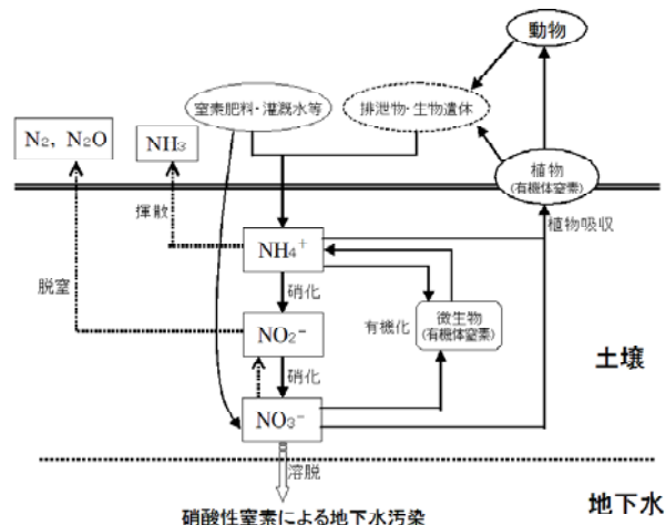
図3-10 土壌中における窒素の動態と地下水汚染模式図
