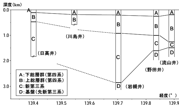
図4-6 深層ボーリングによる推定断面(日高-流山)
