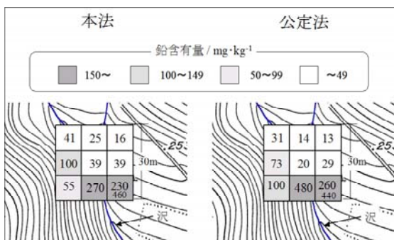
図3-8 射撃場における土壌汚染調査結果
