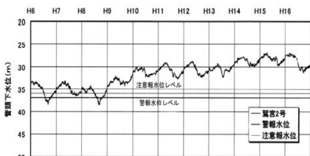
図3-1 鷲宮観測所における最近の地下水水位変化 10)
