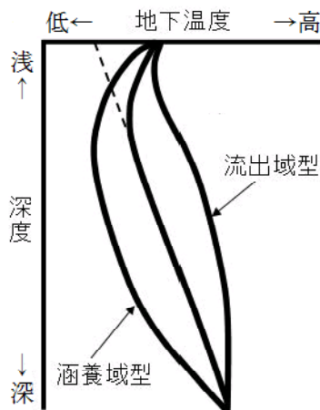
図2-8 地下温度プロファイルの模式図(元図 8) より作成)
