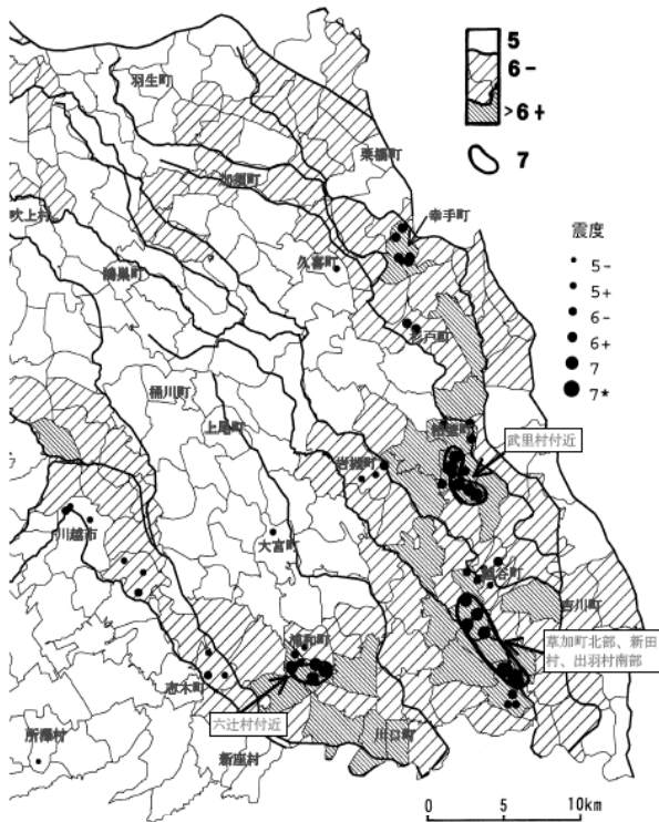
図4-1 被害状況調査報告書から推定した埼玉県東部地域における大正の関東地震の震度分布 17)
