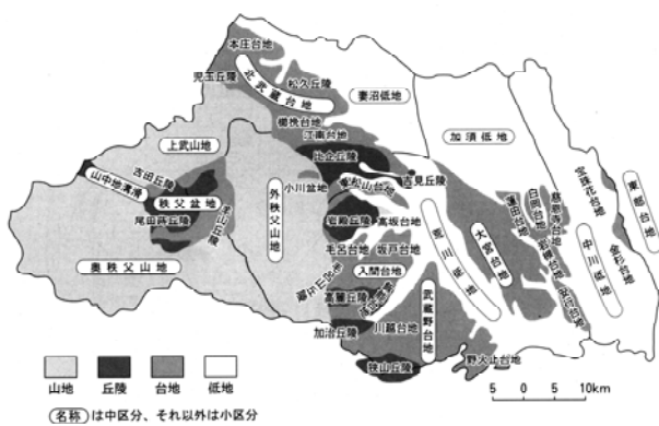
図2-1 埼玉県の地形分類図 1)
