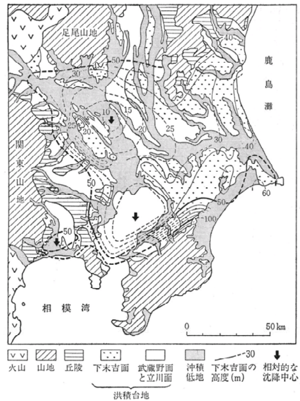
図2-2 関東平野の地形と第四紀後期の地殻変動 2)
