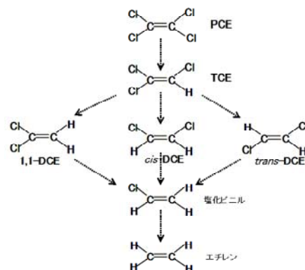
図3-14 PCE及びTCEの理論的還元反応
