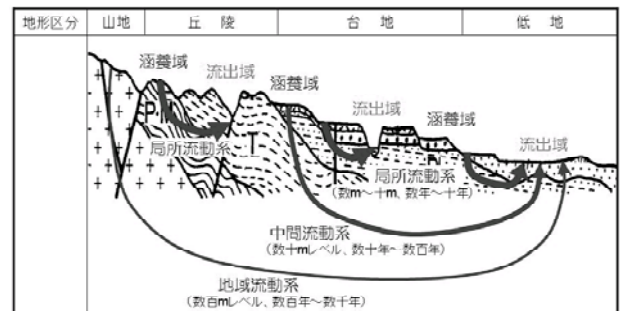
図2-4 地下水循環システムの概念図
