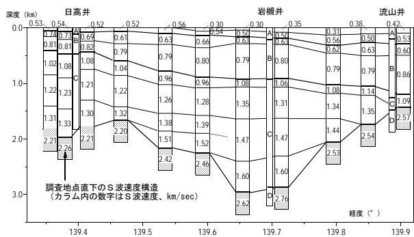
図4-7 S波速度断面(日高一流山) 21)
