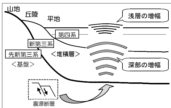
図4-4 地下構造と地震波の伝わり方
