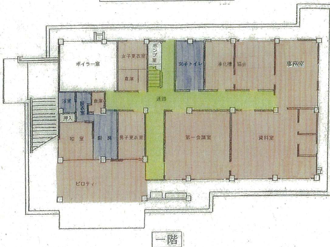
庁舎内配置図 (1/200)
