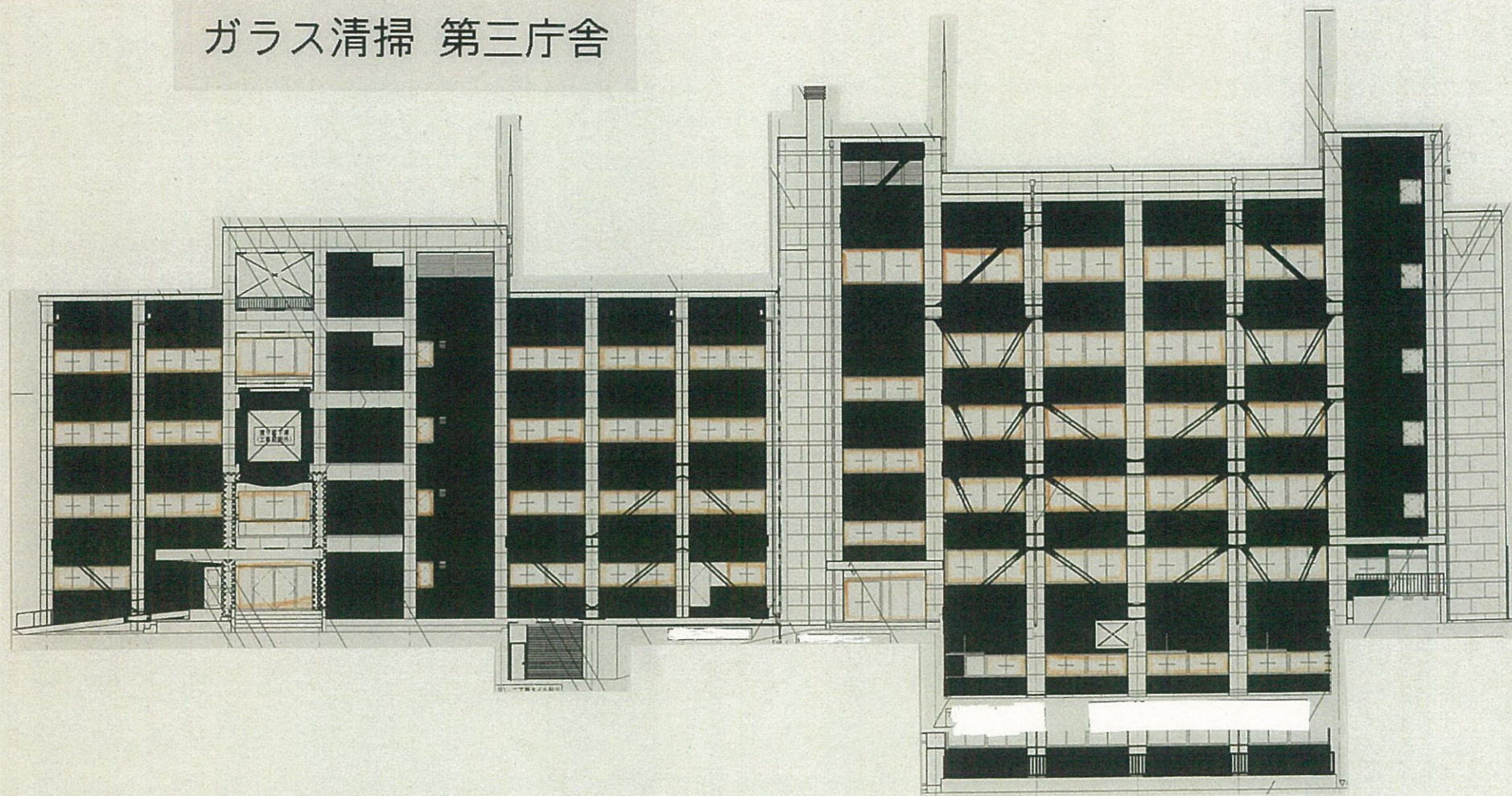
第三庁舎 北立面図
