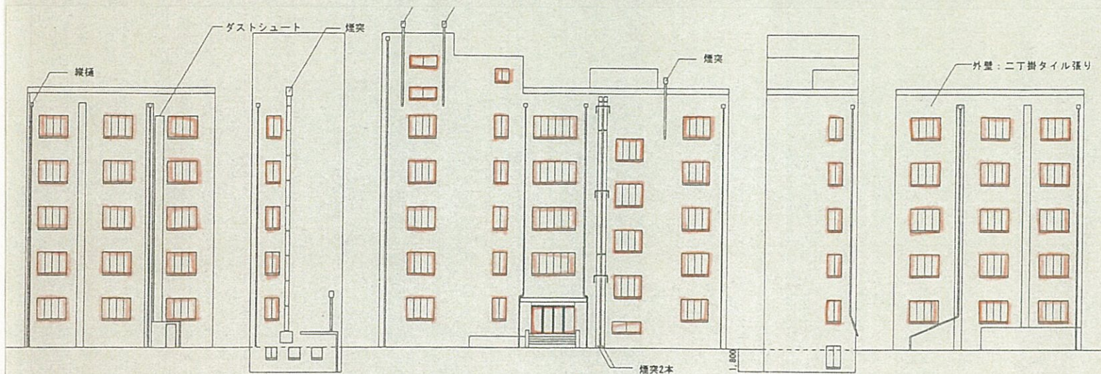
中庭 南面立面図
