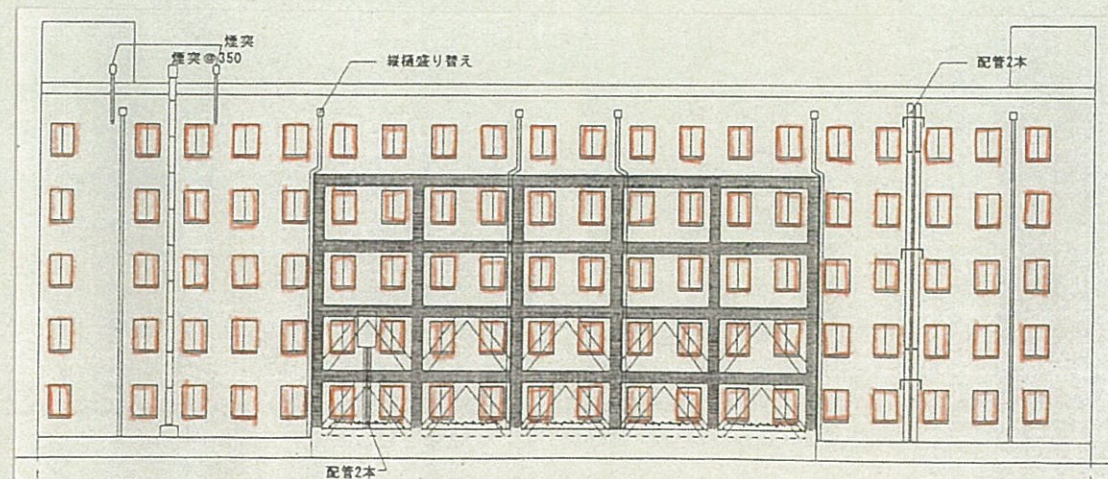
中庭 北面立面図
