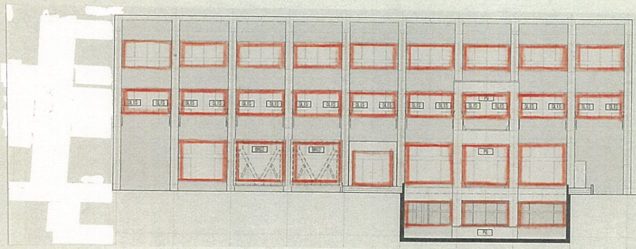
別館 北側立面図
