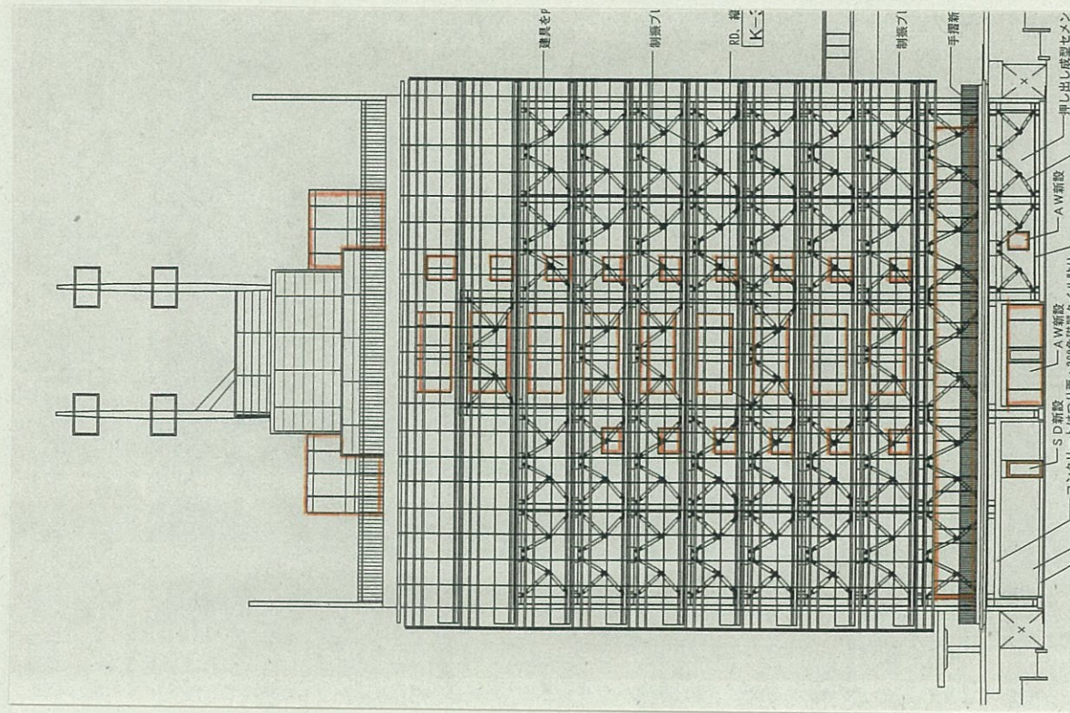
第二庁舎 西側立面図
