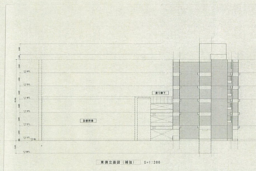
事務所棟 東側立面図
