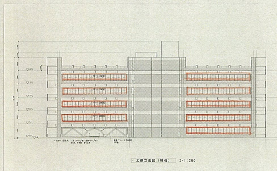
事務所棟 北側立面図
