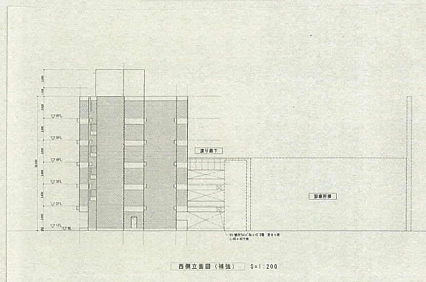
事務所棟 西側立面図
