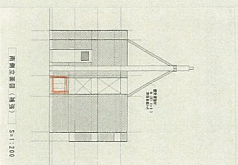
診療所棟 南側立面図
