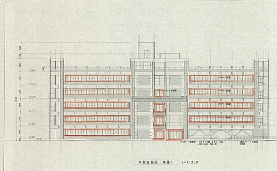
事務所棟 南側立面図
