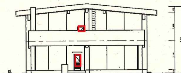
西側立面図 S=1/100
