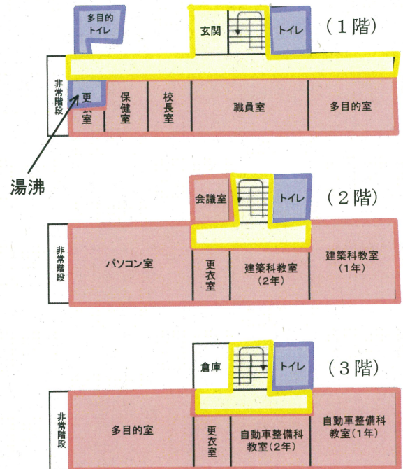
(管理棟平面図)
