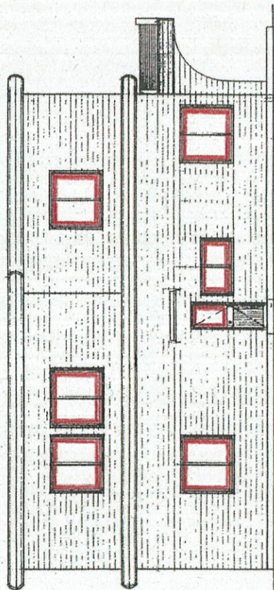
(X 11 ) 東側立面図 S=1/100
