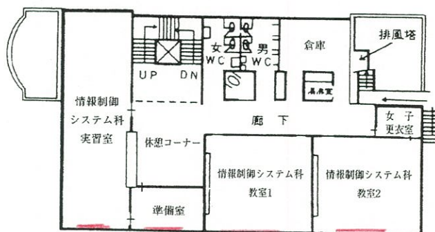
2階平面図
