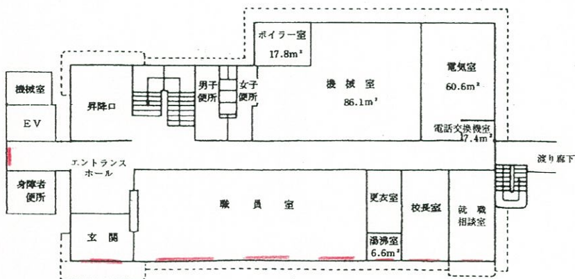
1 階平面図
