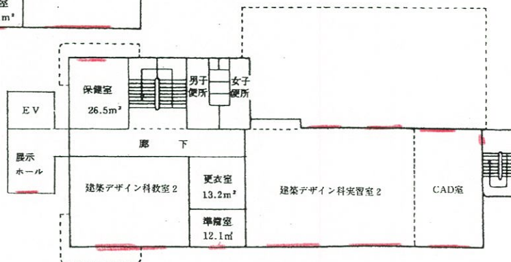
2 階平面図
