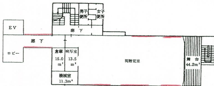
5 階平面図
