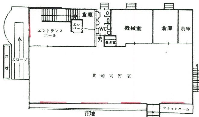
1階平面図
