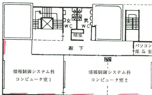
3階平面図
