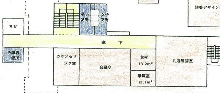
3 階平面図
