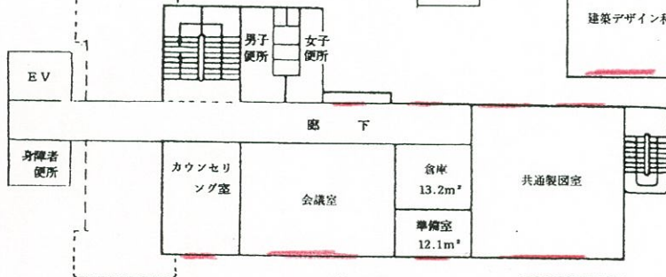
3 階平面図
