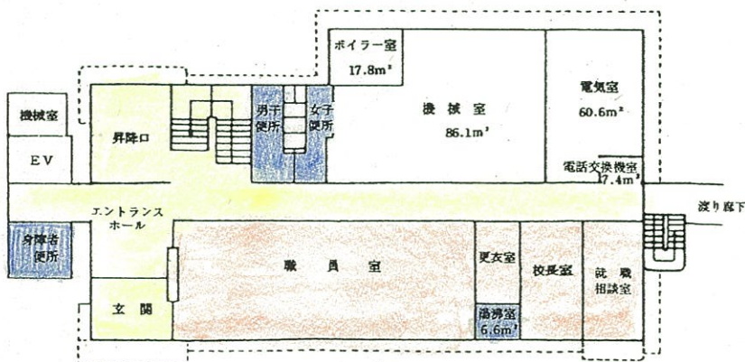
1 階平面図
