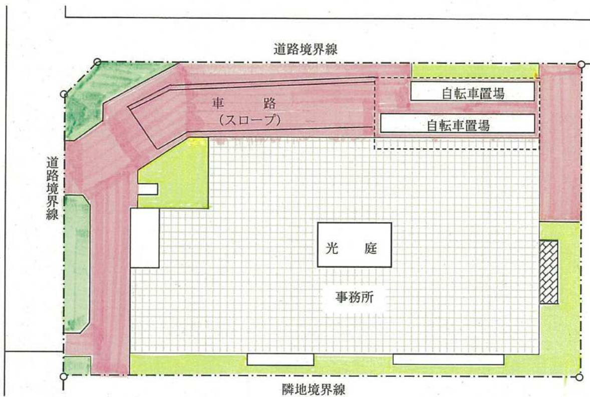
配置図
