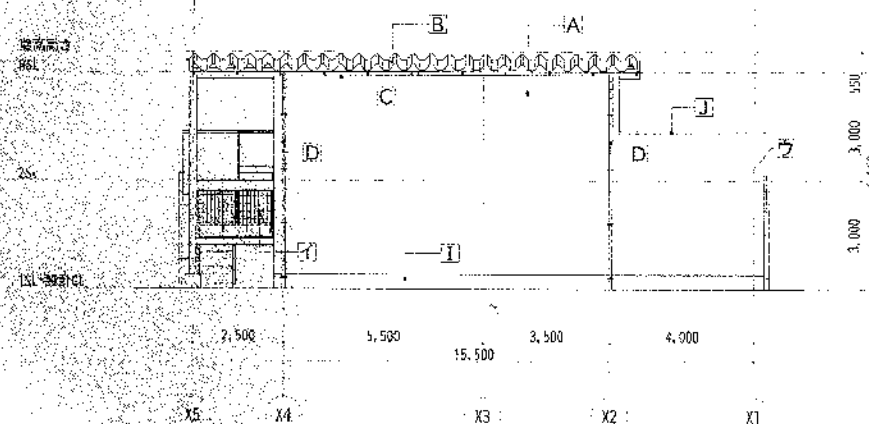
北側立面図
