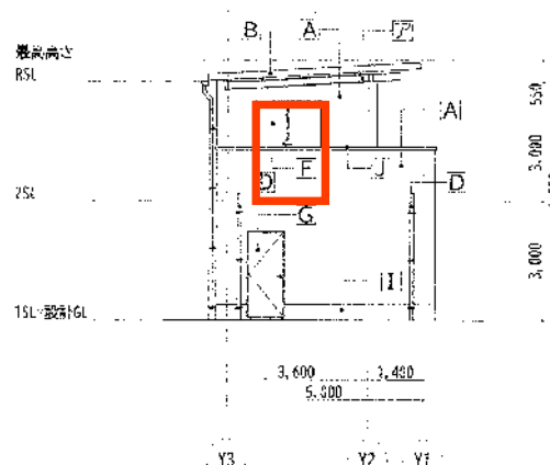
西側立面図
