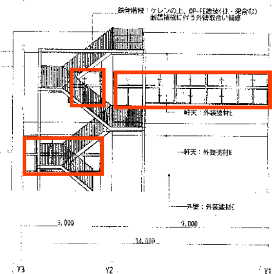
本館 西側立面図 (改修後) 1:100
