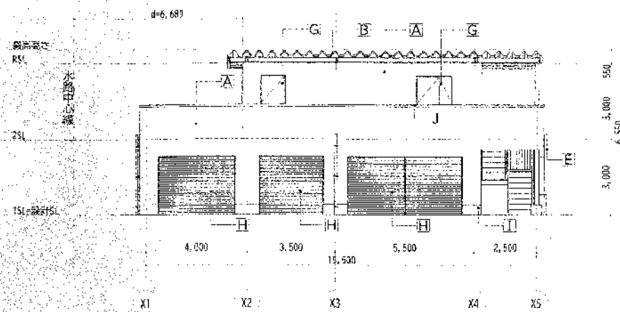
南側立面図
