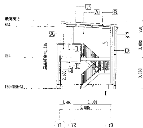
東側立面図
