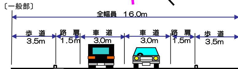
標準横断面
