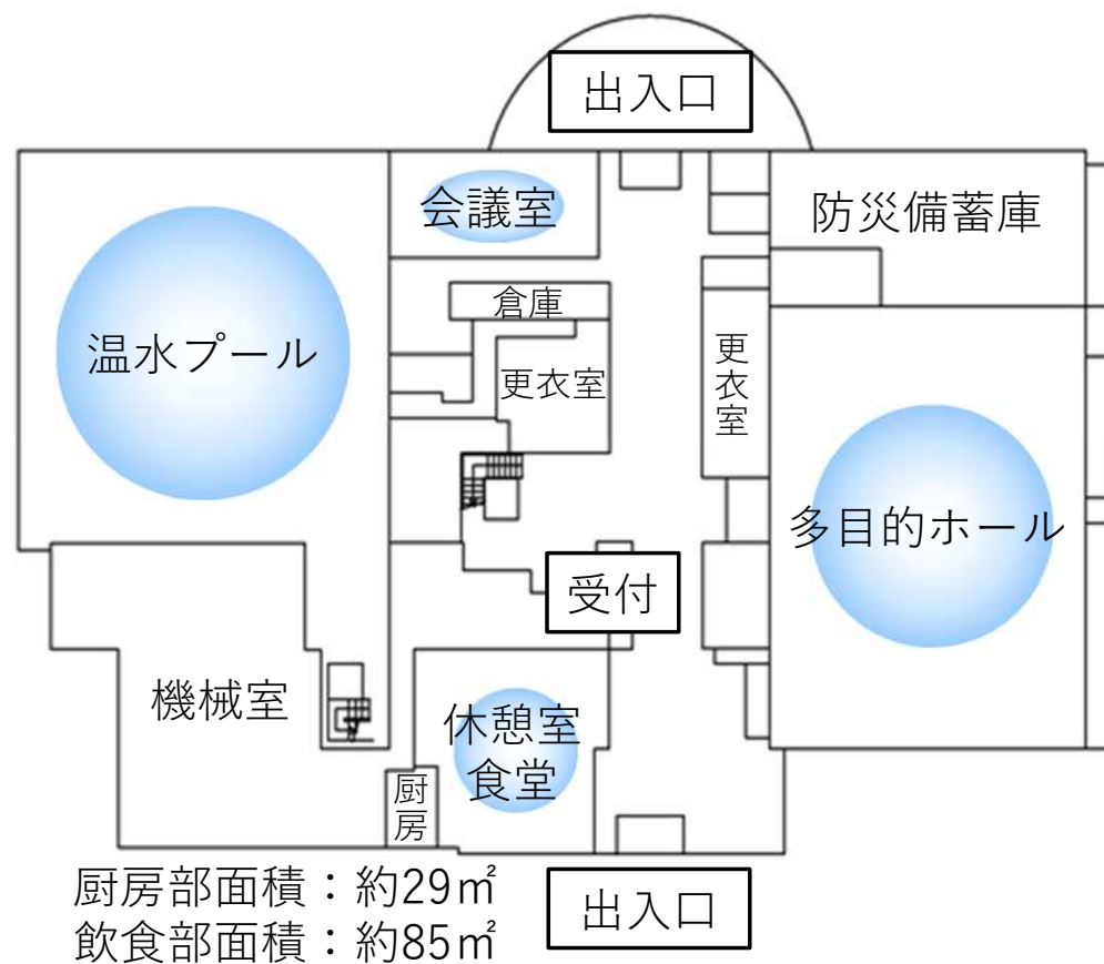
1 階平面図
