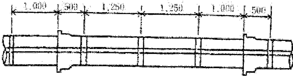
图-2 6m 管
