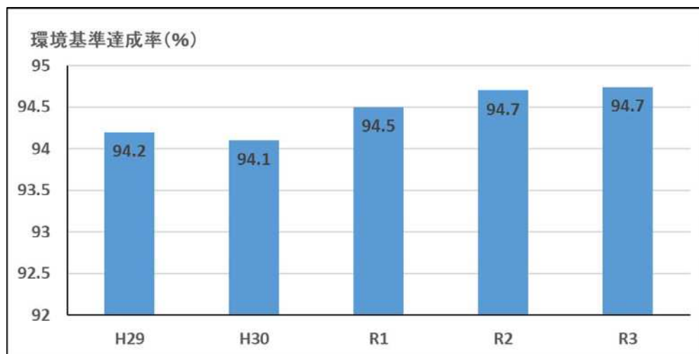
図1 過去の環境基準達成率（面的評価）
