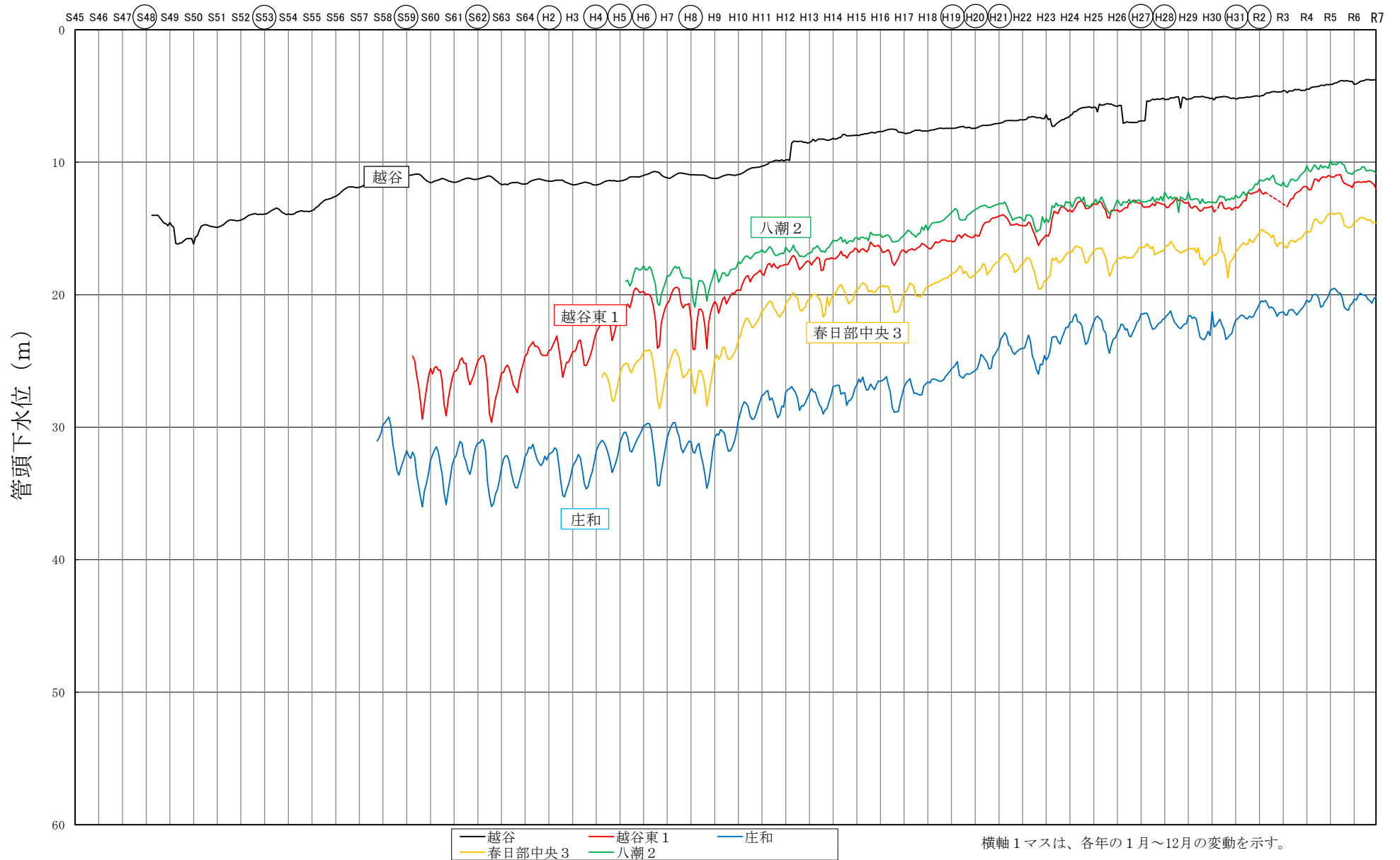
図 1-13 管頭下水位経年変化（東部地域） (○印は湯水年)
