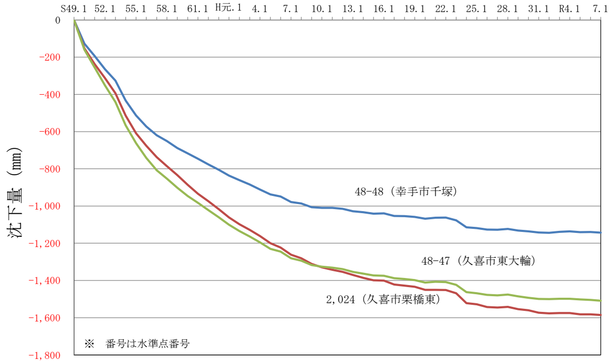
図1-9 地盤沈下経年変化図（幸手市、久喜市）
