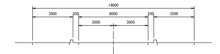
D-D' 断面図
