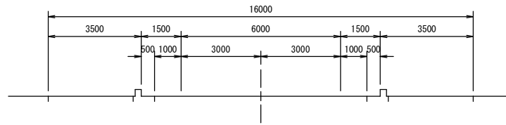
B-B' 断面図
