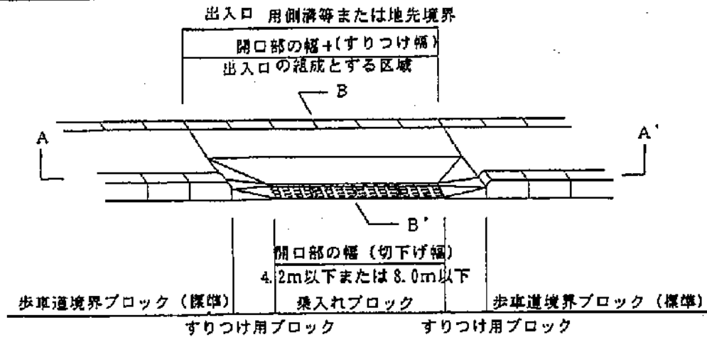
A-A' 断面図
