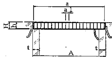
図 7-19 集水ます蓋 (歩行者の通行が考えられる場合は、細目タイプを使用する)
